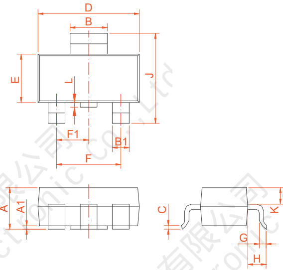
SOT-223-2L
