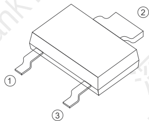
SOT-89-2L
