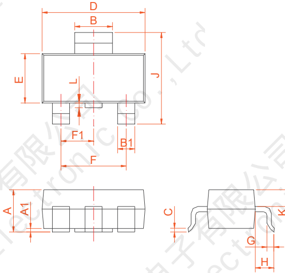
SOT-223-2L
